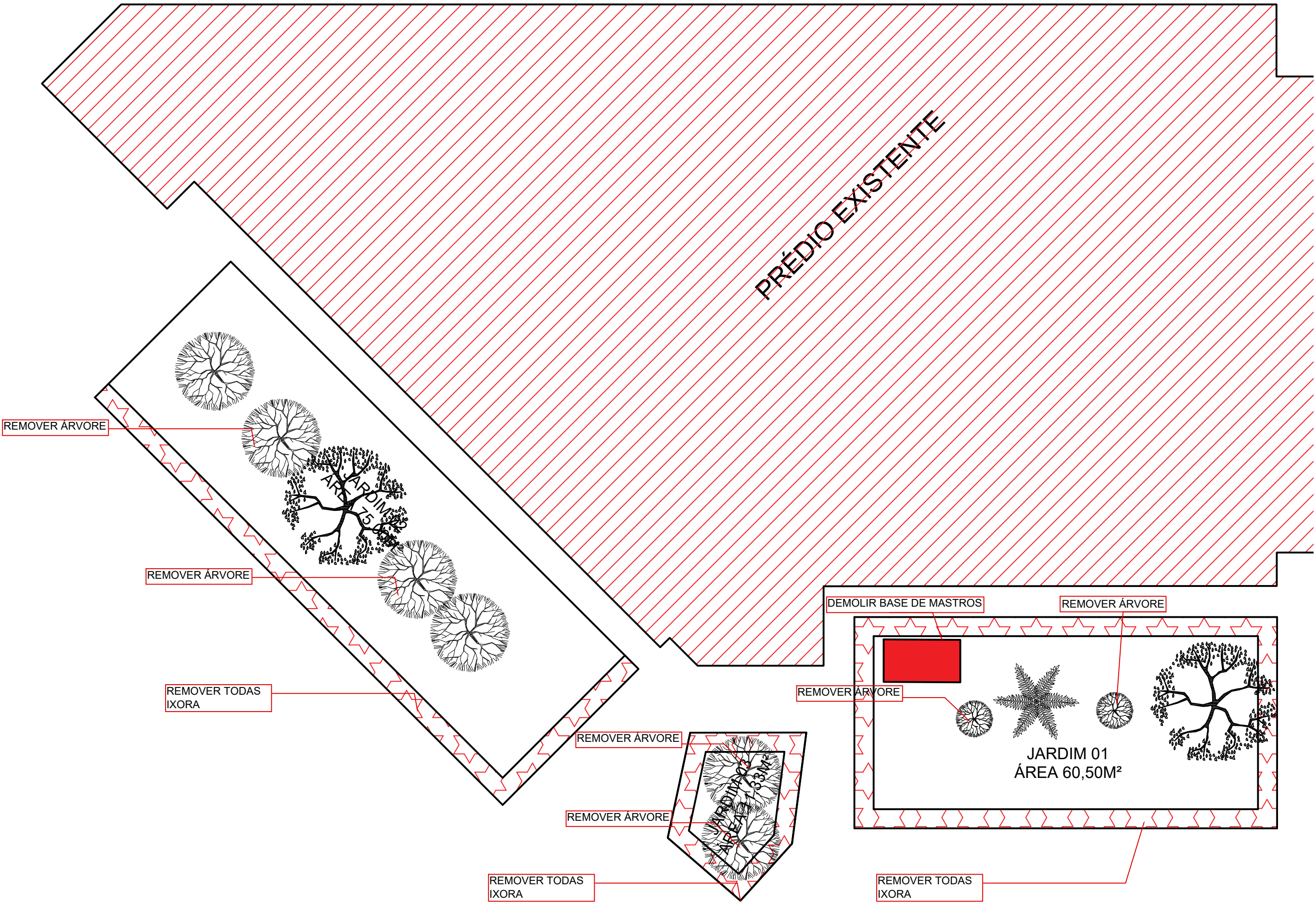
03 Jardim Existente Sem esc.
